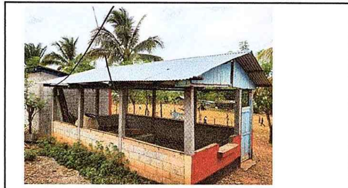
Foto 2: Estructura de madera en mal estado, requiere cambio
